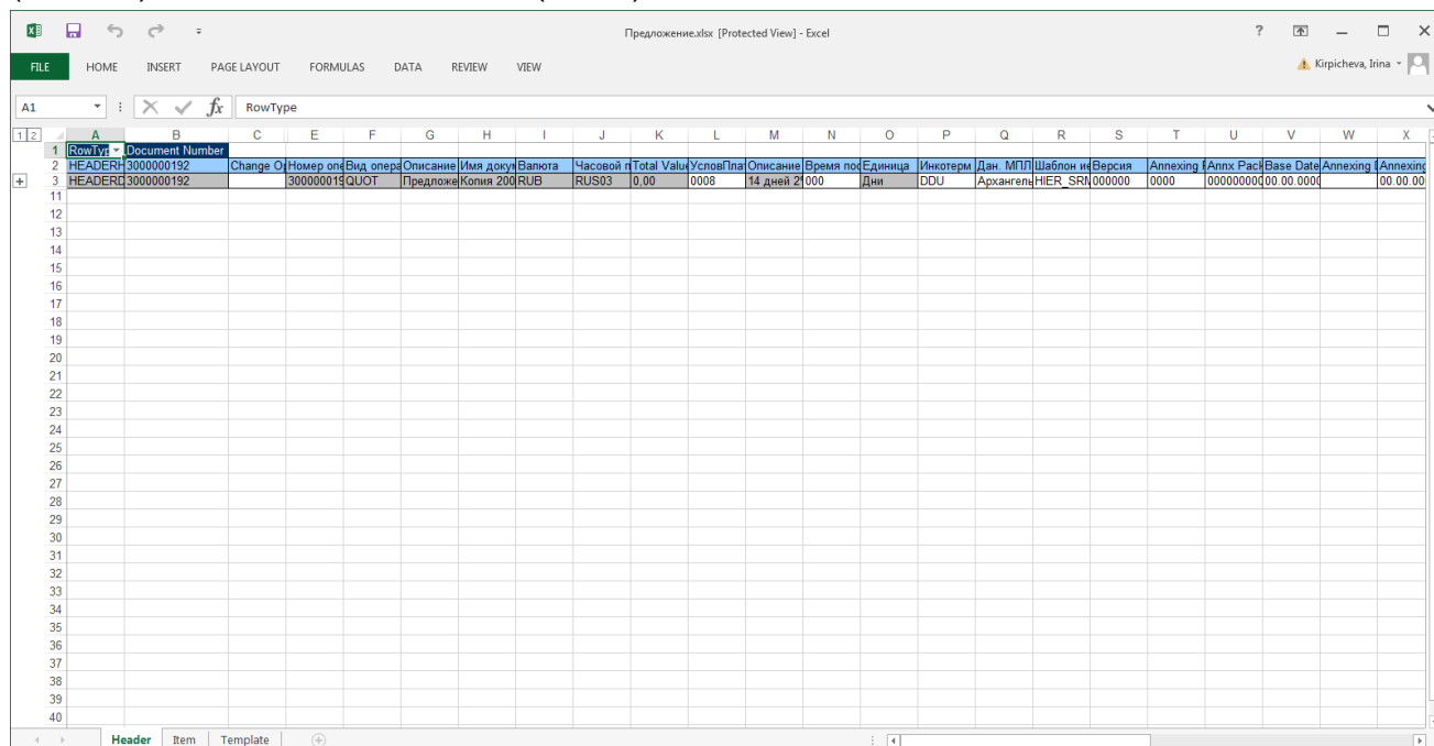
Рисунок 57. Данные заголовка
